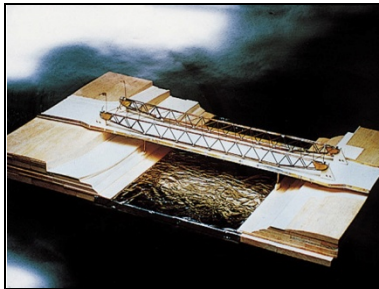
Schönaubücke Graz Projekt 1983
